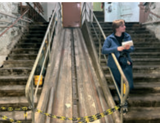
Vår guide vid trappan upp till en 15 cm haubits. Ammunitionshissen i mitten
